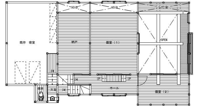
2階平面
