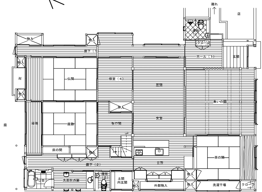
1階平面
