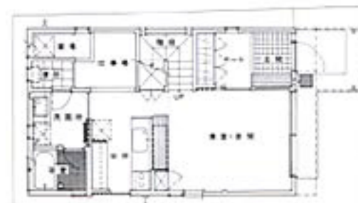
1階平面
